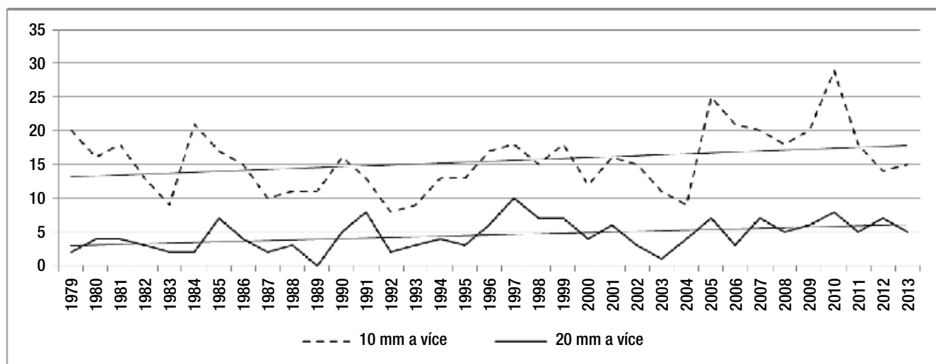
Roční počet dnů se srážkami 10 mm a více a 20 mm a více.
