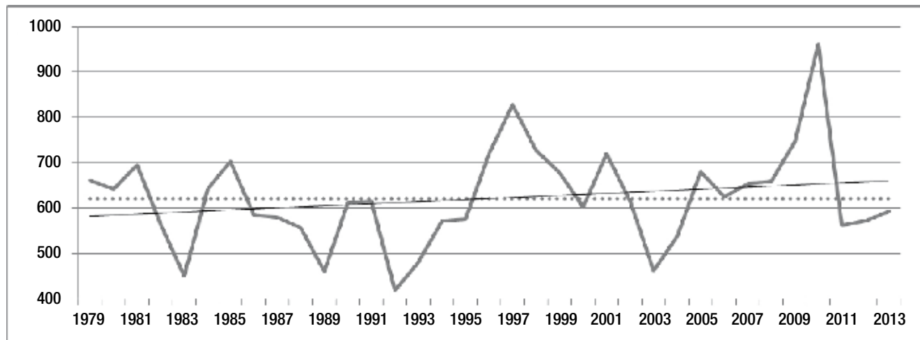
Roční srážkové úhrny a jejich lineární trend.
