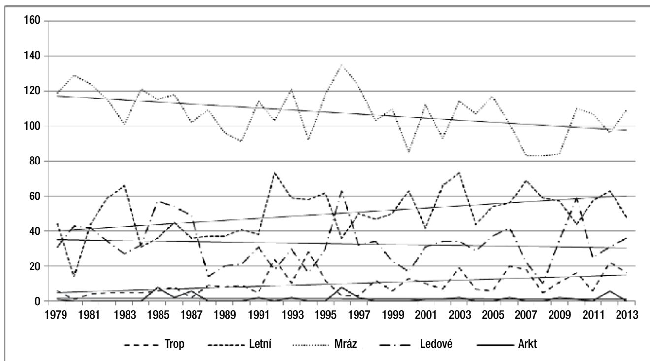
Roční počty charakteristických dnů a jejich lineární trendy.
