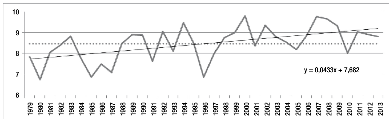
Průměrná roční teplota vzduchu v Hladkých Životicích.
