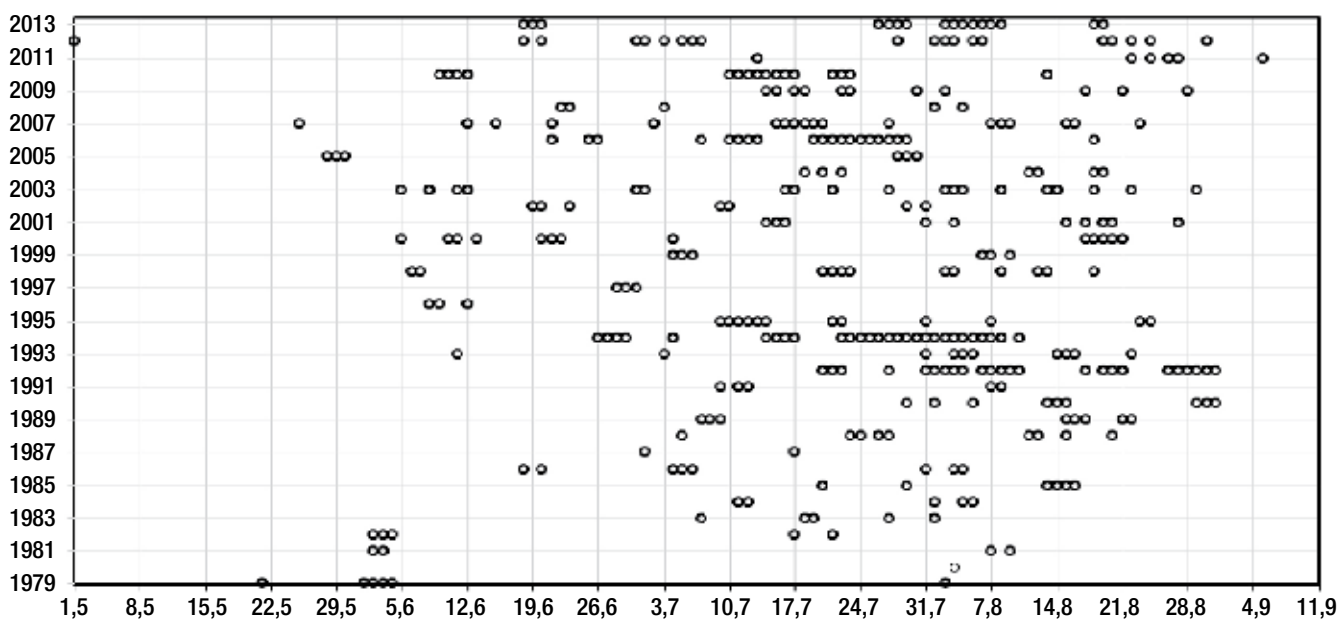
Grafické vyjádření výskytu tropických dnů v jednotlivých rocích.
